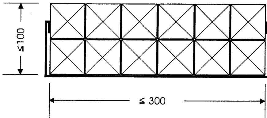
Gruppe von Nachinstallationskeilen in Wandabschottung
